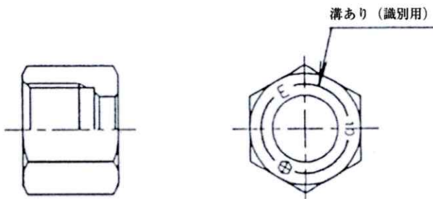
エンベロープ付スリーブ用ナットの識別標示
