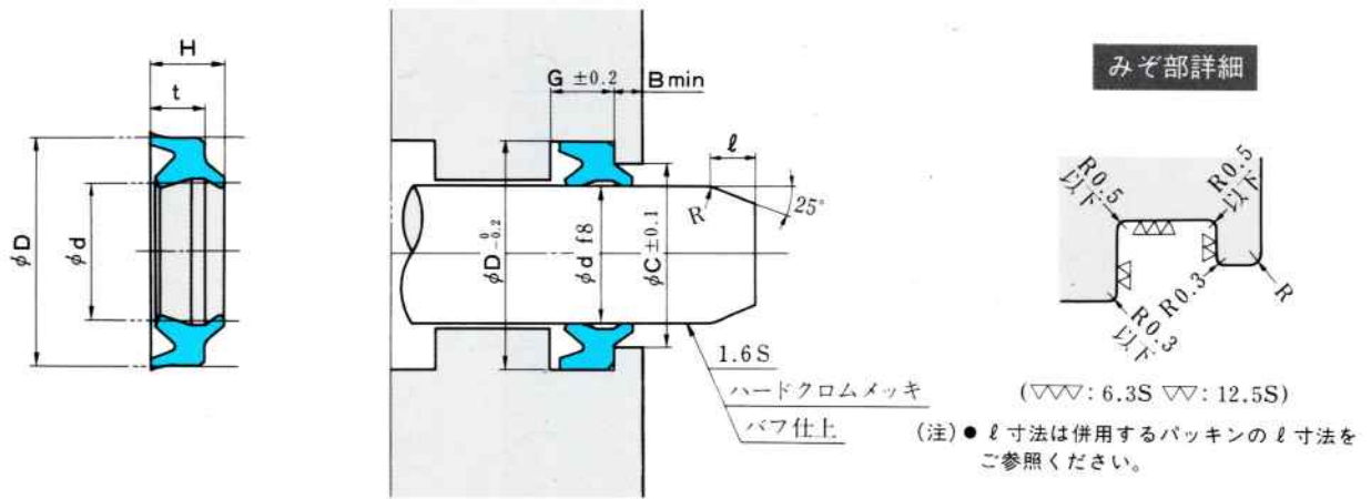
SDRスクレーパ寸法表
