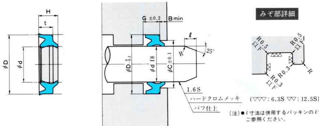
SDRスクレーパ寸法表
